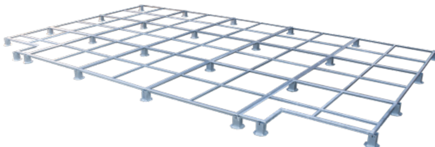
» STELAŻ POD ZESKOK / MODULAR GRID PLATFORM FOR LANDING AREA
